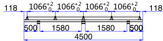
横レールの取付図
