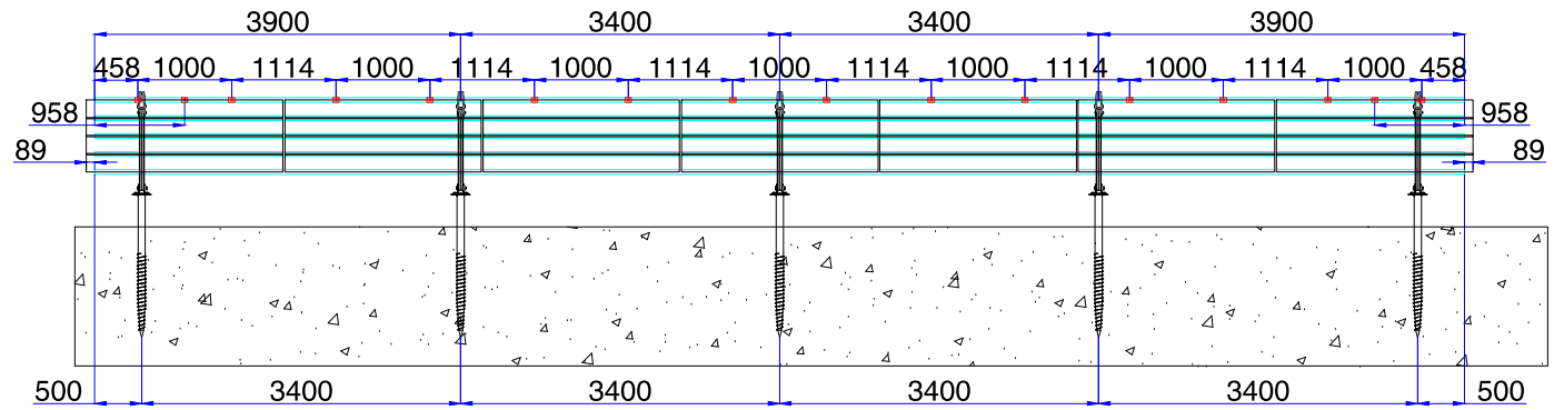
横レール寸法、スパン (E/W) 図
