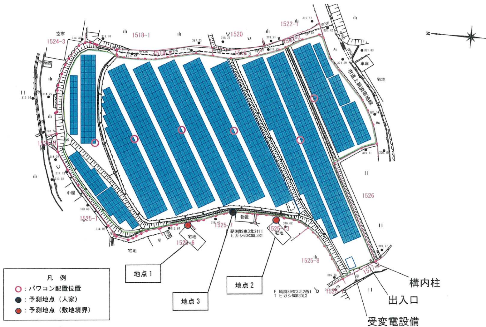
図 5-1-2 設備機器の稼働位置及び予測地点
